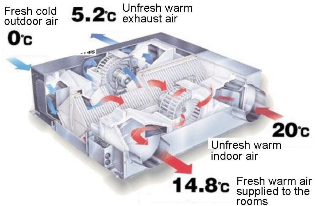
Figura 11 Principiul de funcționare al recuperatorului.
