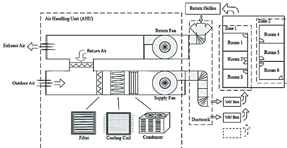
Figura 4. Unitate de tratare a aerului (AHU) [7]
