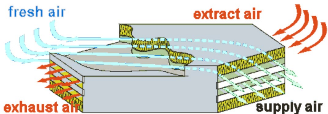
Figur 12 Prinsippskisse av en platevarmeveksler.
