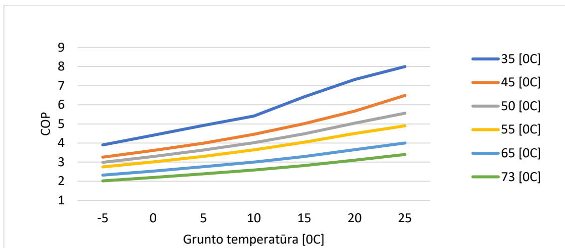
12 pav. COP kitimas priklausomai nuo žemės temperatūros.
