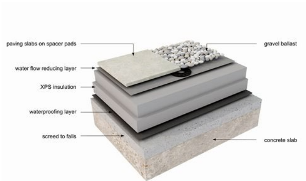
Figura 10: Cubierta plana
