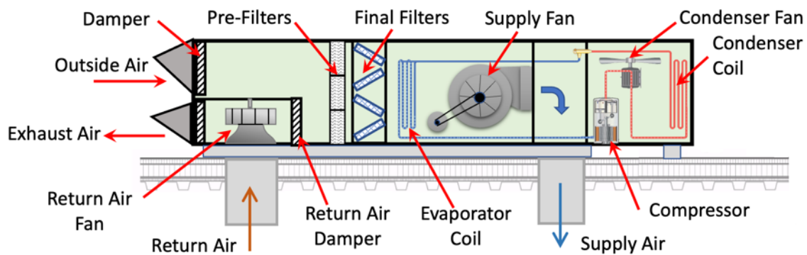
Figur 11. Pakkesystemer [12]
