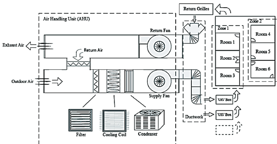
Figur 4. Luftbehandlingsenhet (AHU) [7]
